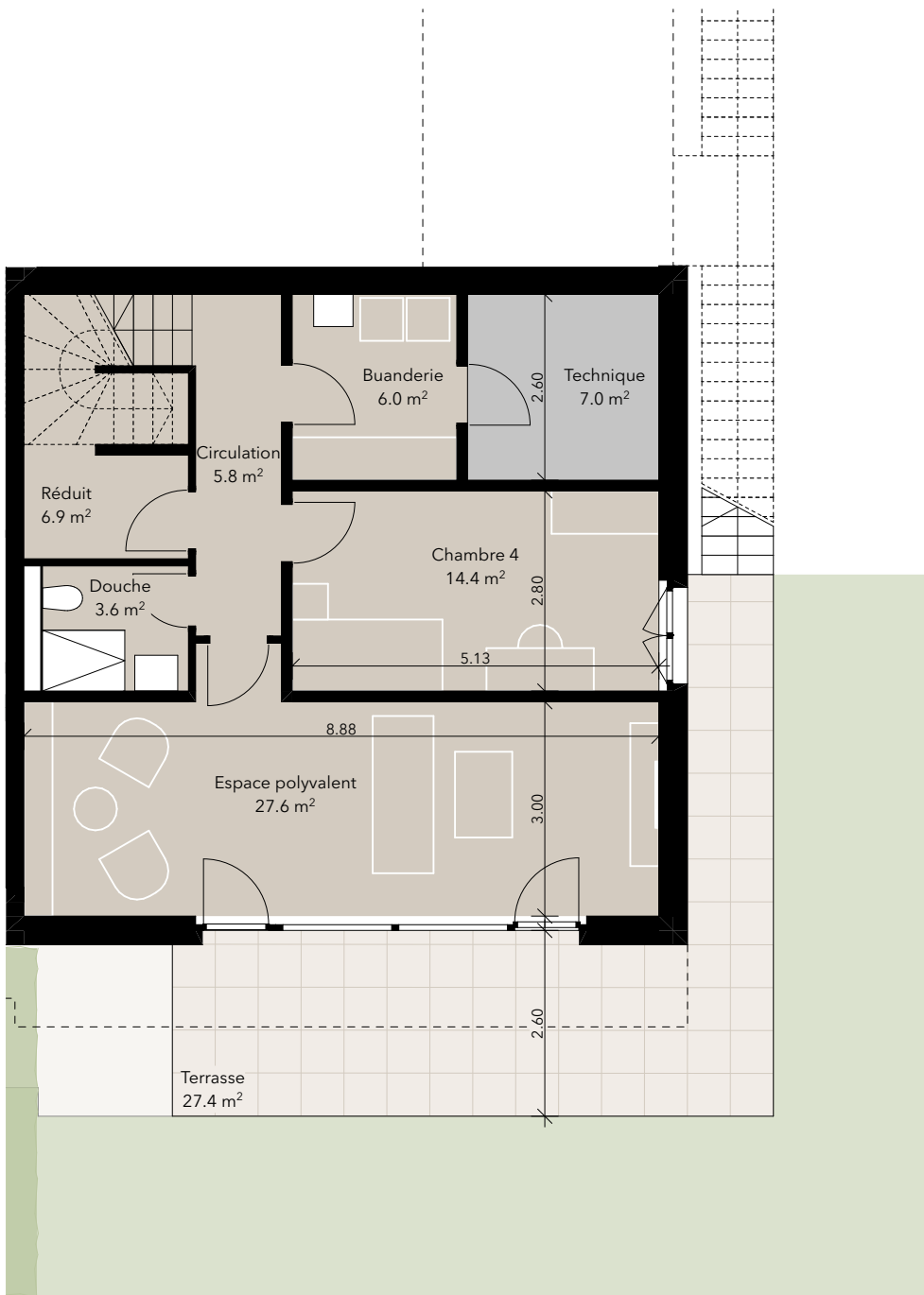
VILLA A2 - NIVEAU 0 (Jardin)
